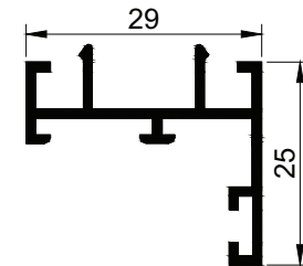
3022 m = 0,413 \text{ kg/m}
