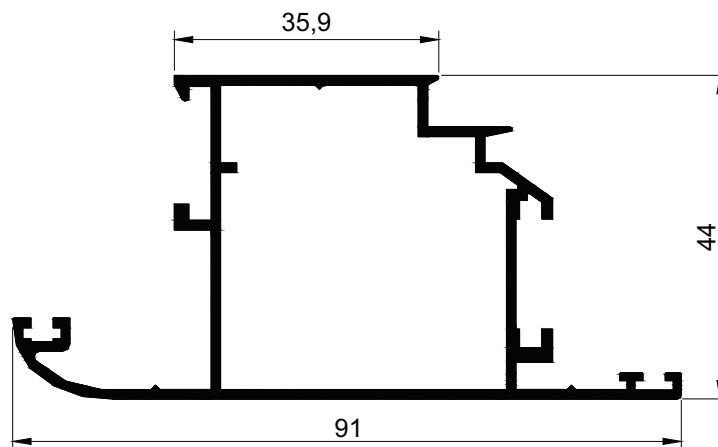
3814 m = 0,956 \text{ kg/m}
