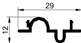
3027 m = 0,289 \text{ kg/m}
