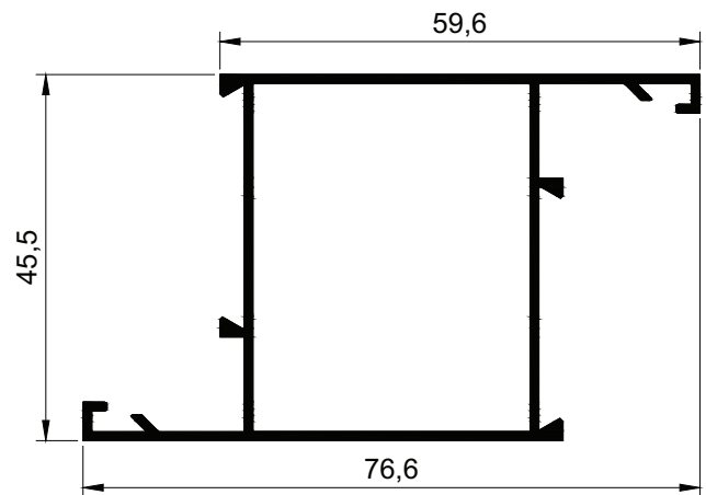
3075 m = 0,771 kg/m
