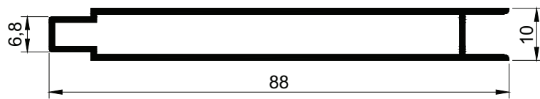
3010 m = 0,614 kg/m
