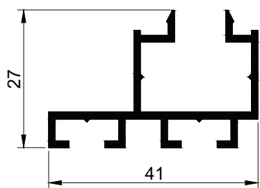
3553 m = 0,463 \text{ kg/m}
