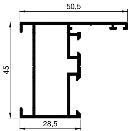
3622 m = 0,679 \text{ kg/m}
