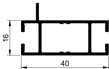
3313 m = 0,492 kg/m
