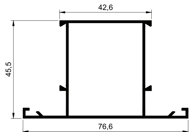
3074 m = 0,771 kg/m
