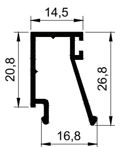
3419 m = 0,249 \text{ kg/m}
