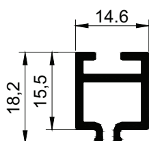
2071 m = 0,252 \text{ kg/m}
