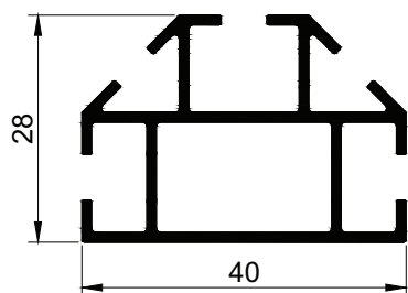
3581 m = 0,606 kg/m
