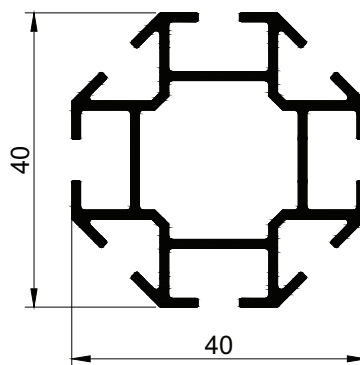
3582 m = 0,770 kg/m
