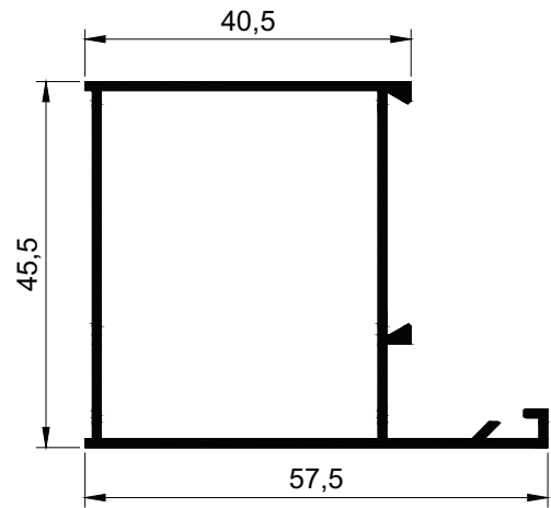
3073 m = 0,650 kg/m
