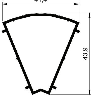
3810 m = 0,458 \text{ kg/m}
