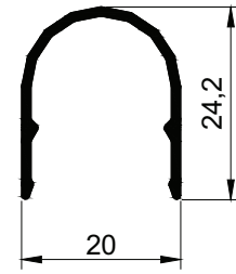
3067 m = 0,306 \text{ kg/m}
