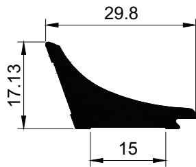
6025 m = 0,471 kg/m
