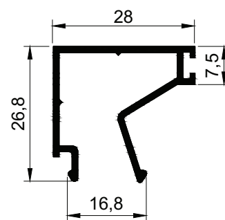
3399 m = 0,328 \text{ kg/m}
