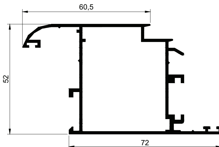
3420 m = 1,202 kg/m
