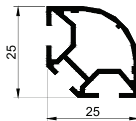
3314 m = 0,398 kg/m
