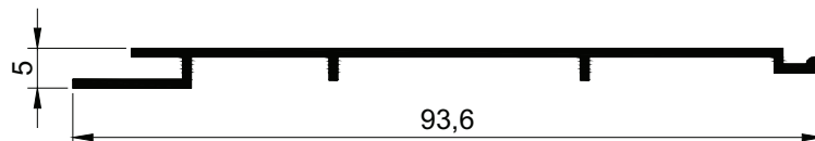
3012 m = 0,365 kg/m
