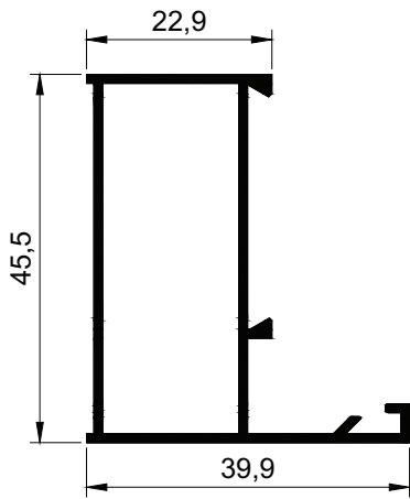
3080 m = 0,536 kg/m
