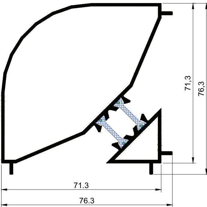
3474 m=1,436 kg/m
