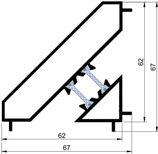
3473 m=1,284 kg/m
