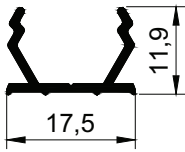
3068 m = 0,106 \text{ kg/m}
