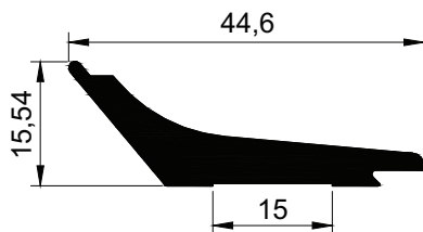
6027 m = 0,610kg/m
