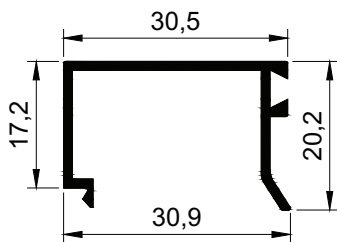
3009 m = 0,246 kg/m
