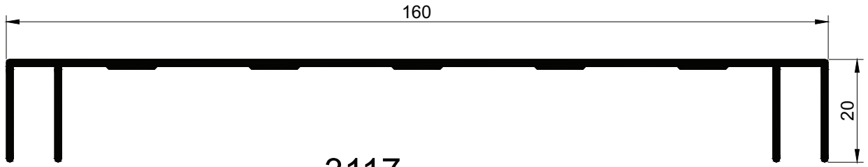
3117 m = 0,948 \text{ kg/m}
