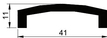
6022 m = 0,473 \text{ kg/m}
