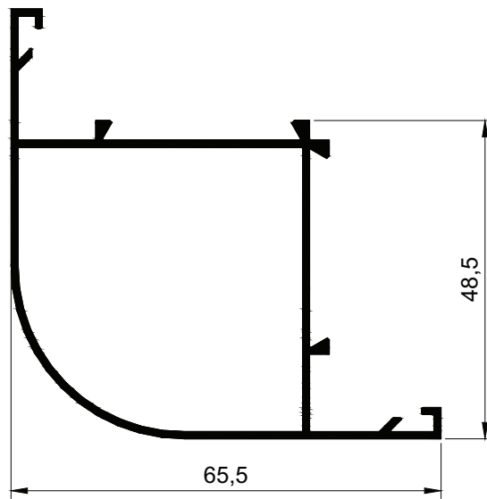
3908 m = 0,777 kg/m
