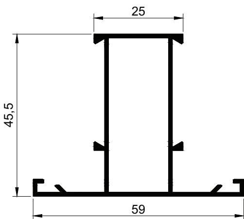
3078 m = 0,656 kg/m
